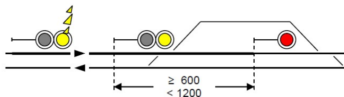
Ingresso in binario di corretto tracciato e fermata in stazione quando la distanza fra il segnale di protezione e il segnale di partenza sia uguale o superiore a m. 600 e inferiore a m. 1200
