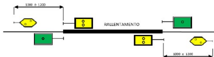
Rallentamento su linea a semplice binario
